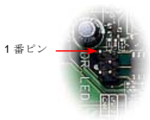
Dr. LED コネクタ
