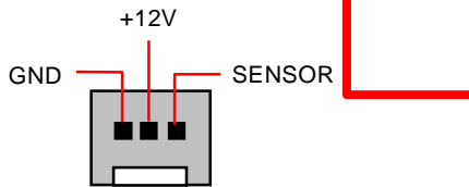
筐体ファンコネクタ
