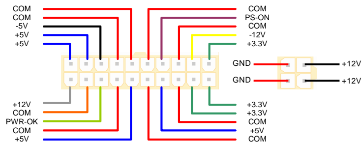
5V/3.3V 外部電源コネクタ
