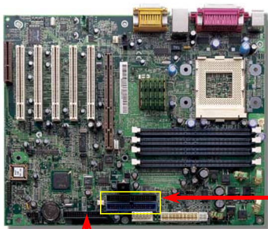
ATA 33/66/100 IDE コネクタ
