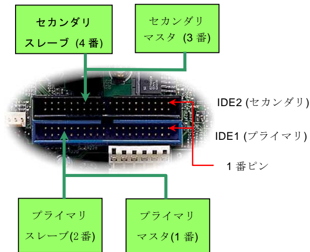
ATA 33/66/100 IDE コネクタ
