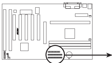
IDE Connectors
