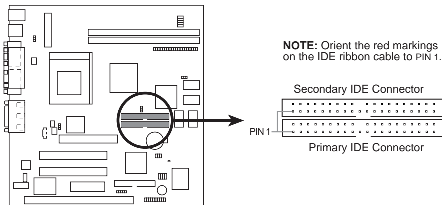
MEZ-VM IDE Connectors
