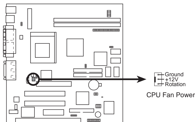
MEZ-VM Cooling Fan Connector
