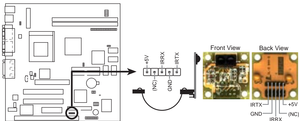
MEZ-VM Infrared Module Connector
