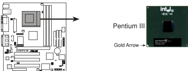
CUEP2-M Socket 370
