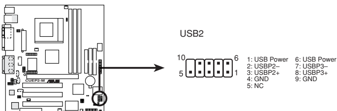
CUEP2-M USB Headers
