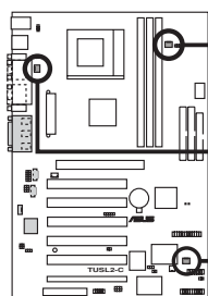
TUSL2-C 12-Volt Cooling Fan Power
