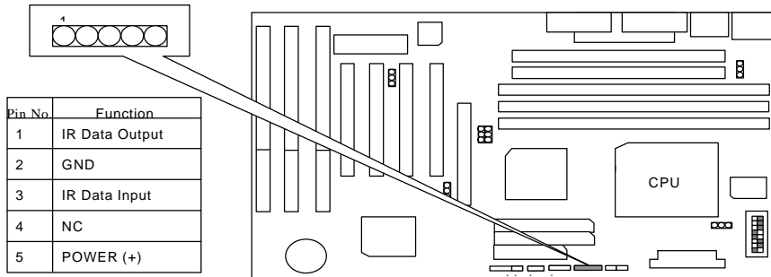
GN : Green Function Switch
